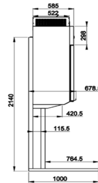
GANIMED XL TOP P&P
